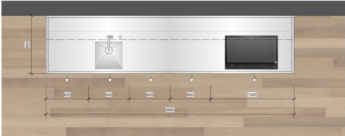
Grundriss
